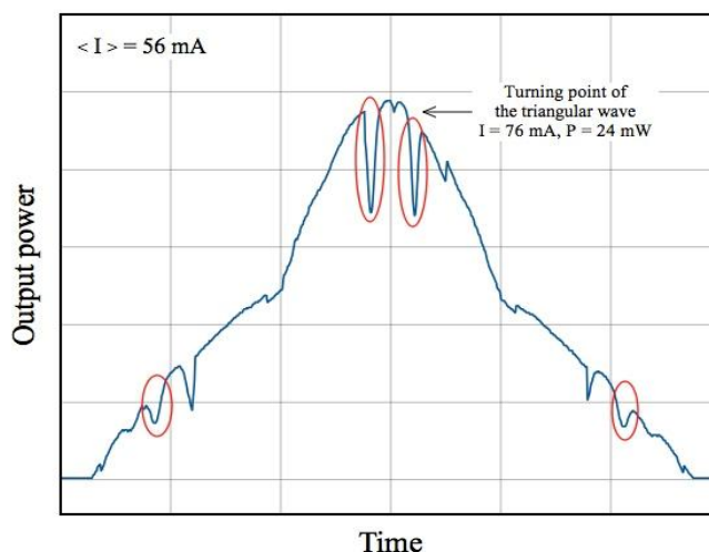
Рис. 3. Зависимость выходной мощности лазера от тока инжекции. Ток лазерного диода модулируется симметричным треугольным сигналом. Красные эллипсы обозначают зону поглощения лазерного излучения в парах Cs.
