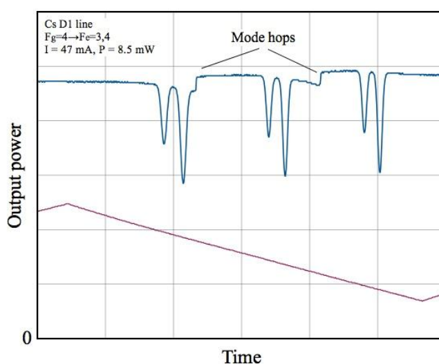
Рис. 4. Зависимость выходной мощности лазера на выходе из Cs ячейки от напряжения на пьезоэлементе (синяя кривая). Напряжение меняется линейно со временем (модулирующий сигнал приведен ниже красным). Ток лазерного диода не меняется.
