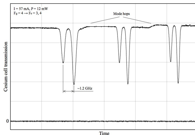
Рис.4. Зависимость выходной мощности лазера на выходе из Cs ячейки от напряжения на пьезоэлементе. Напряжение меняется линейно со временем (показан только один склон модулирующего сигнала). Ток лазерного диода не меняется.
