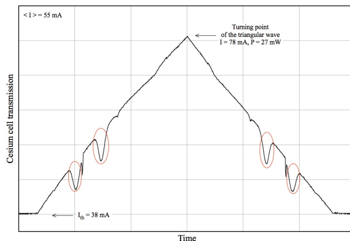
Рис.3. Зависимость выходной мощности лазера от тока инжекции. Ток лазерного диода модулируется симметричным треугольным сигналом. Зависимость снята при постоянном напряжении на пьезоэлементе. Красные эллипсы выделяют зоны поглощения лазерного излучения в парах Cs.
