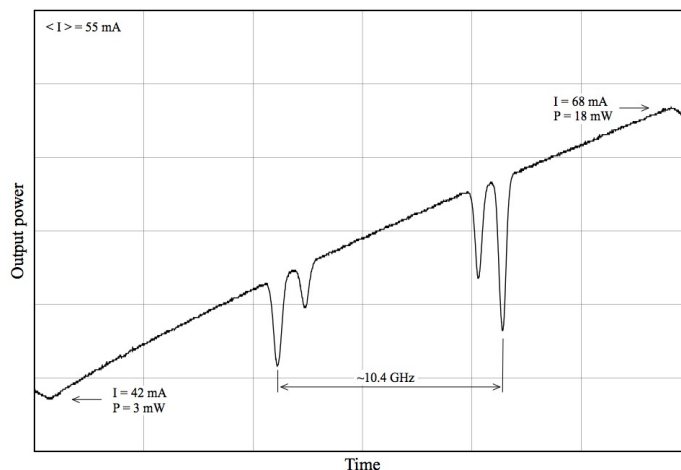
Рис.5. Пропускание ячейки с парами Cs при синхронном сканировании дифракционной решетки и тока ЛД.
