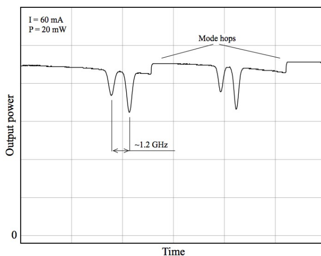
Рис.4. Зависимость выходной мощности лазера на выходе из Cs ячейки от напряжения на пьезоэлементе. Напряжение меняется линейно со временем (показан только один склон модулирующего сигнала). Ток лазерного диода не меняется.
