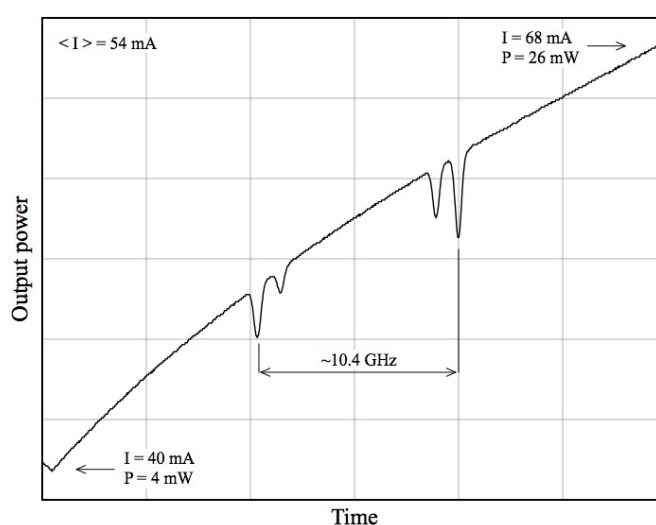
Рис.5. Пропускание ячейки с парами Cs при синхронном сканировании дифракционной решетки и тока ЛД.
