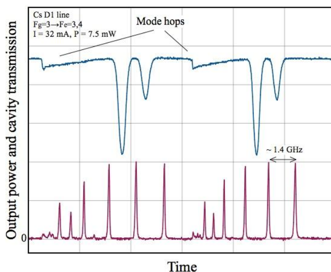
Рис. 4. Зависимости выходной мощности лазера на выходе из Cs ячейки (верхняя синяя кривая) и пропускания конфокального интерферометра (нижняя красная кривая) от напряжения на пьезоэлементе. Напряжение меняется линейно со временем (показан только один склон модулирующего сигнала). Ток лазерного диода не меняется.
