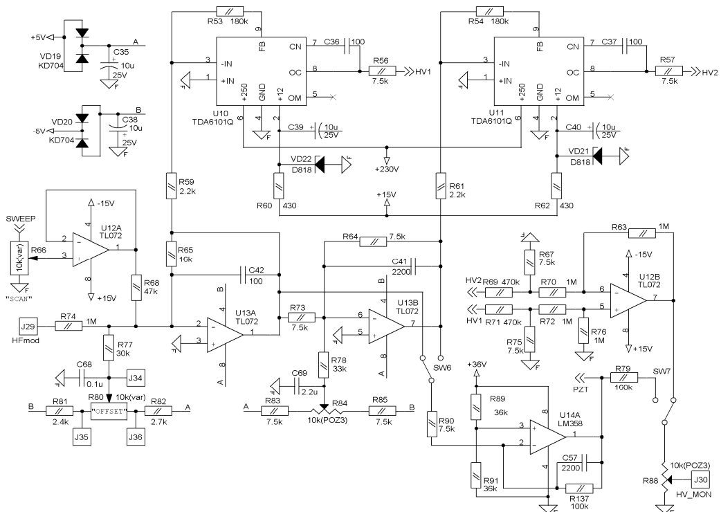
Рис.10. Схема высоковольтного усилителя.
