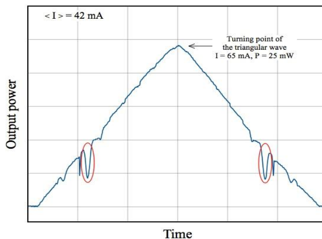
Рис. 3. Зависимость выходной мощности лазера от тока инжекции. Ток лазерного диода модулируется симметричным треугольным сигналом. Красные эллипсы обозначают зону поглощения лазерного излучения в парах Cs.
