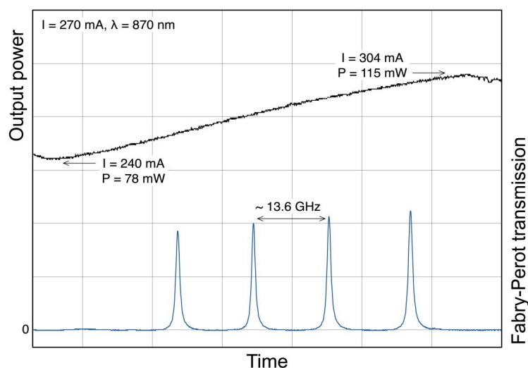
Рис.5. Мощность ECDL-8750R (верхняя кривая) и пропускание эталона Фабри-Перо (нижняя кривая) при синхронном сканировании дифракционной решетки и тока ЛД.
