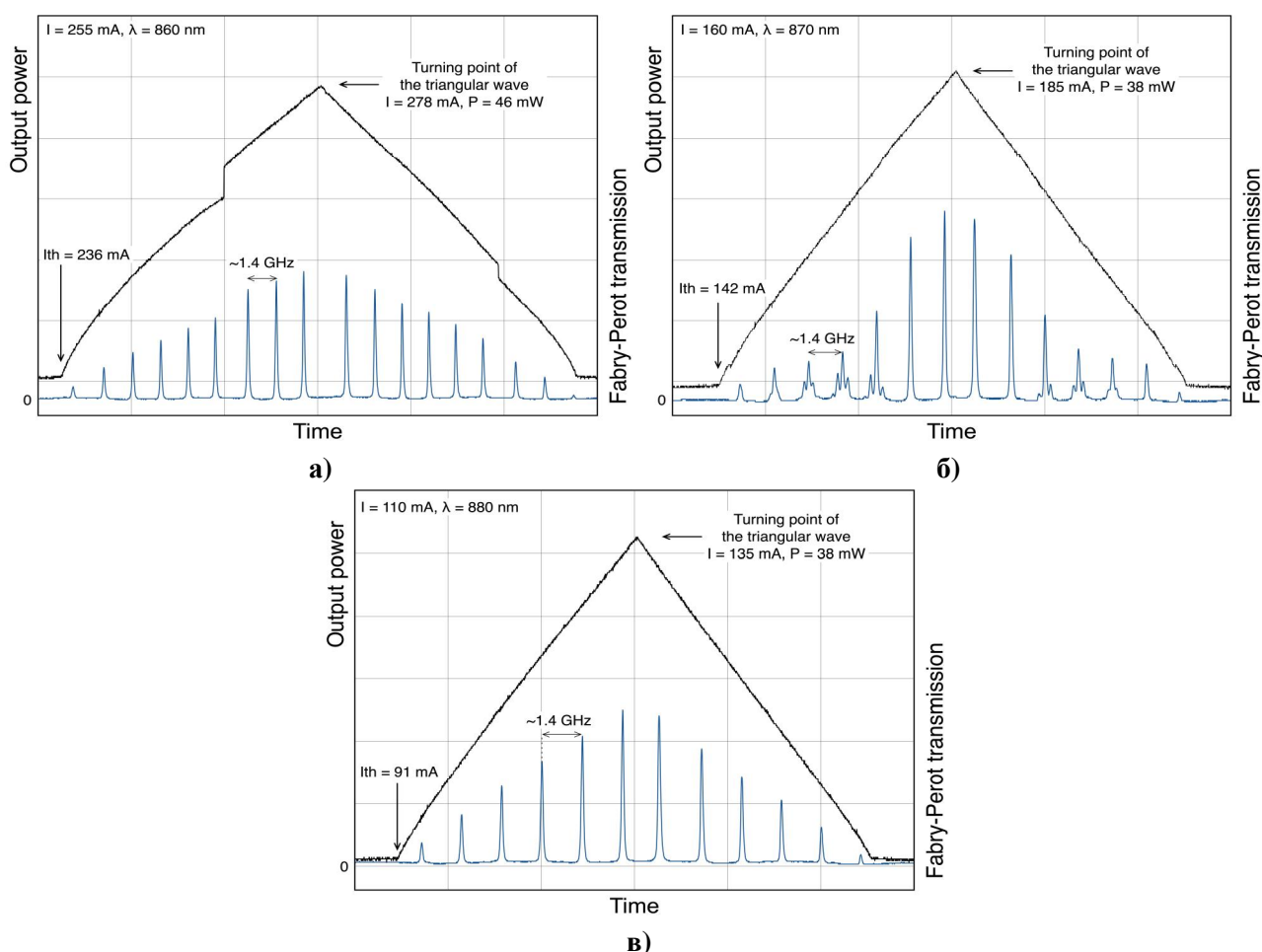
Рис.3. Зависимости выходной мощности лазера от тока инжекции для разных длин волн (верхние черные кривые). Ток лазерного диода модулируется симметричным треугольным сигналом. Зависимости сняты при постоянном напряжении на пьезоэлементе. Нижние кривые показывают пропускание конфокального интерферометра.
