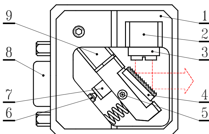
Рис.1. Оптическая головка (вид сверху при снятой крышке). 1 – корпус оптической головки; 2 – хладагентный лазерного диода; 3 – единый модуль лазерного диода и коллимирующего объектива; 4 – дифракционная решетка, укрепленная на горизонтальном валу; 5 – вертикальный фиксирующий винт M2; 6 – горизонтальный юстировочный винт M3x0,25; 7 – пьезоэлемент; 8 – разъем DHS-15F; 9 – подвижный рычаг.
