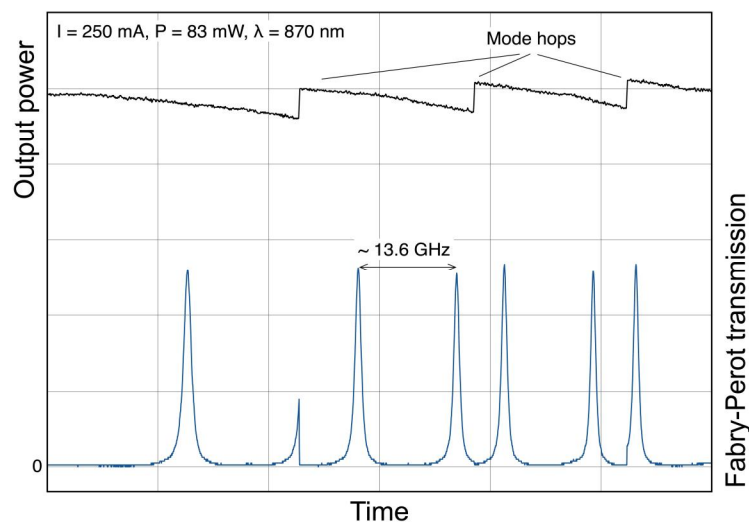
Рис.4. Зависимость выходной мощности лазера от напряжения на пьезоэлементе при постоянном токе LD (верхняя черная кривая). Внизу – пропускание эталона Фабри-Перо с областью свободной дисперсии 13,6 ГГц. Напряжение меняется линейно со временем (показан только один склон модулирующего сигнала), ток лазерного диода не меняется.
