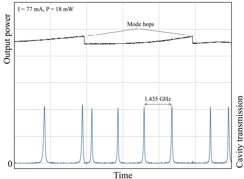
Рис.4. Зависимость выходной мощности лазера от напряжения на пьезоэлементе при постоянном токе LD (черная кривая). Синим – пропускание конфокального интерферометра.
