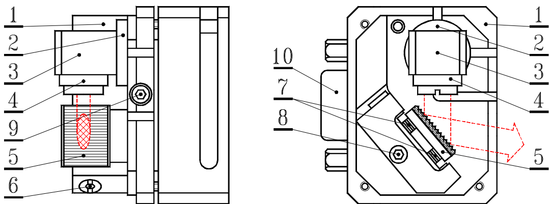
Рис.1. Оптическая головка (вид сбоку и сверху при снятой крышке). 1 – корпус оптической головки; 2 – вертикальный вал; 3 – хладапровод лазерного диода; 4 – единый модуль лазерного диода и коллимирующего объектива; 5 – дифракционная решетка, укрепленная на горизонтальном валу; 6 – горизонтальный вал; 7 – пьезоэлементы; 8 – вертикальный фиксирующий винт M2; 9 – горизонтальный фиксирующий винт M2; 10 – разъем DHS-15F.
