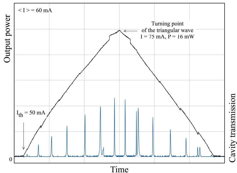
Рис.3. Зависимость выходной мощности лазера от тока инжекции (черная кривая). Ток лазерного диода модулируется треугольным сигналом. Зависимость снята при постоянном напряжении на пьезоэлементе. Синим показано пропускание конфокального интерферометра, имеющего FSR=1435 МГц.
