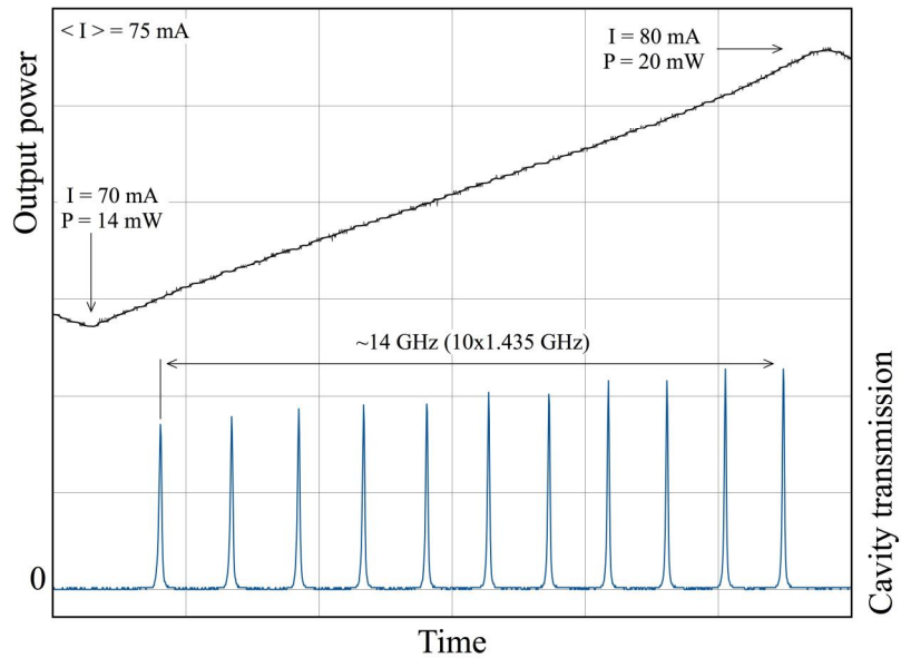
Рис.5. Мощность ECDL-7820 (черная кривая) и пропускание конфокального интерферометра (синяя кривая) при синхронном сканировании пьезоэлемента и тока накачки.
