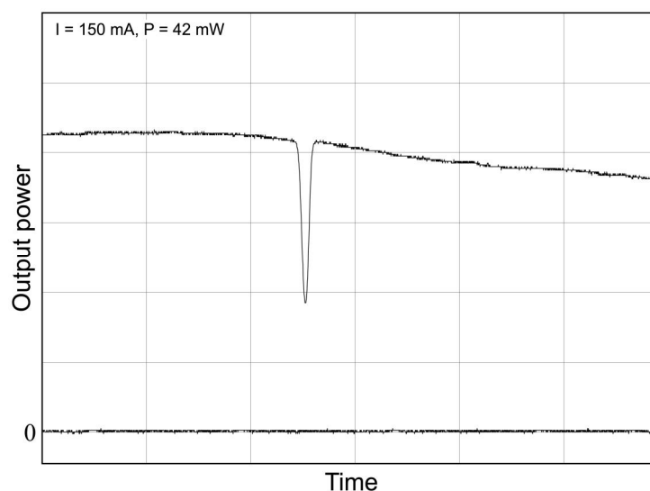
Рис.4. Зависимость мощности лазера на выходе из калиевой ячейки от напряжения на пьезоэлементе. Напряжение меняется линейно со временем (показан только один склон модулирующего сигнала), ток лазерного диода не меняется.
