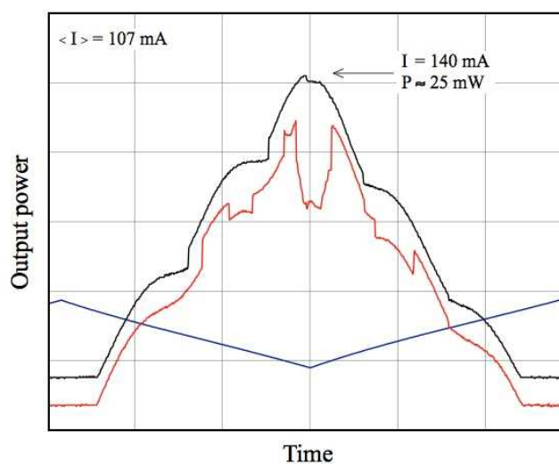
Рис. 3. Зависимости выходной мощности лазера от тока инжекции при различных положениях решетки в плоскости дифракции. Ток лазерного диода модулируется симметричным треугольным сигналом (показан синим цветом). Зависимости сняты при постоянном напряжении на пьезоэлементе.
