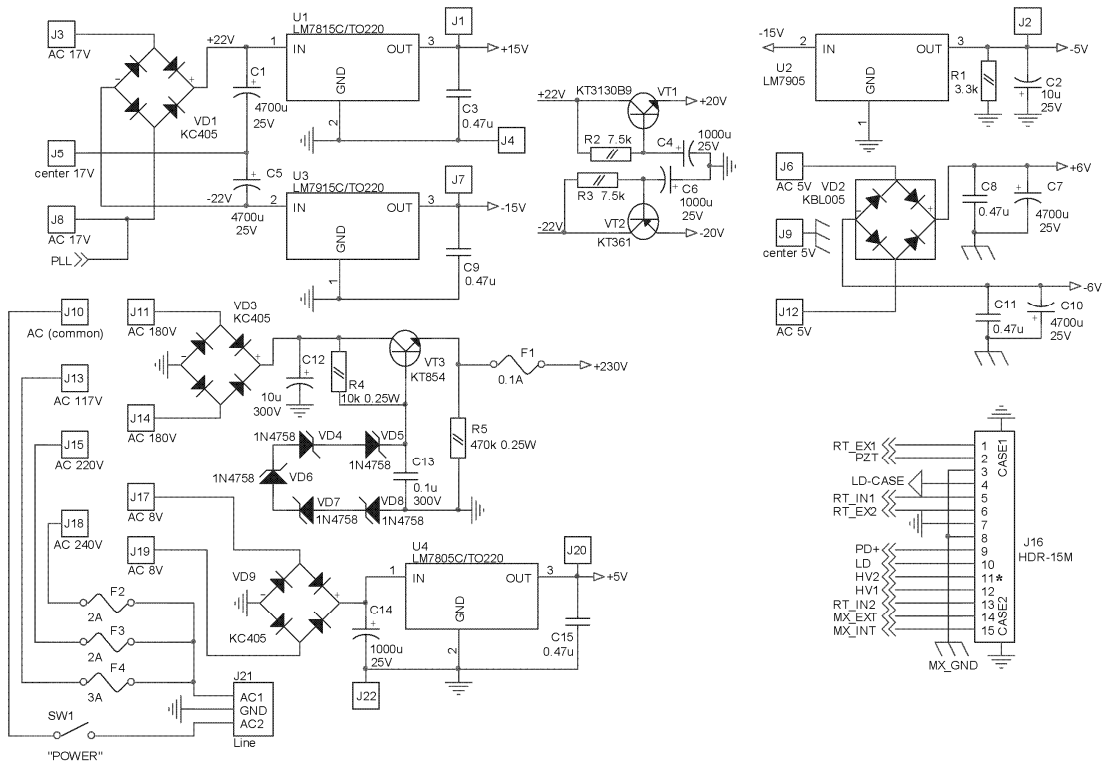
Рис.7. Схема блока питания.
