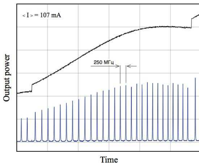
Рис. 4. Зависимости выходной мощности лазера (вверху) и пропускания конфокального интерферометра (внизу) от тока инжекции. Среднее значение тока составляет 107 мА.
