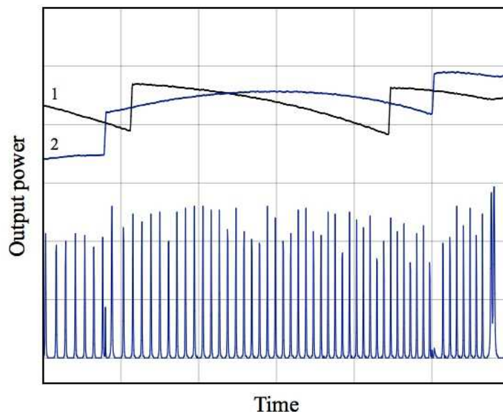
Рис. 6. Мощность ECDL-6720R при сканировании только пьезоэлементов (кривая 1) и пьезоэлементов совместно с током накачки (кривая 2). Внизу приведено пропускание интерферометра соответствующее случаю 2. Флуктуации амплитуды резонансов связаны с оцифровкой сигнала.
