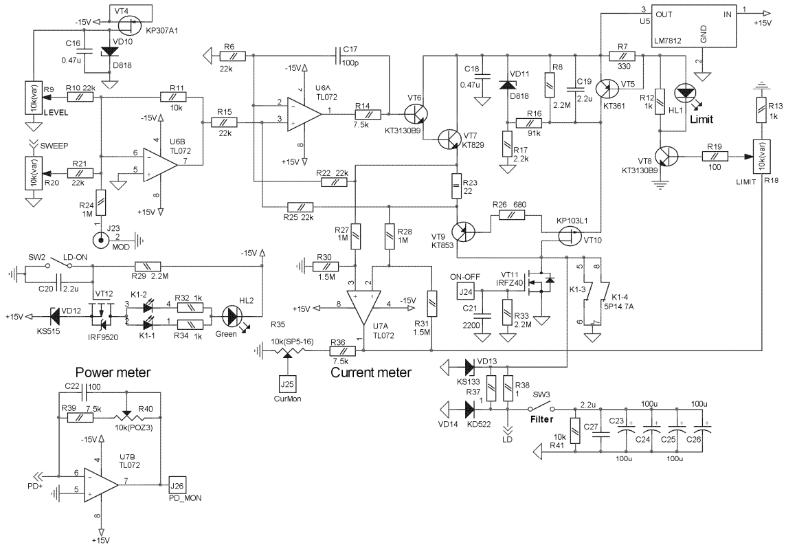
Рис.8. Схема источника тока.
