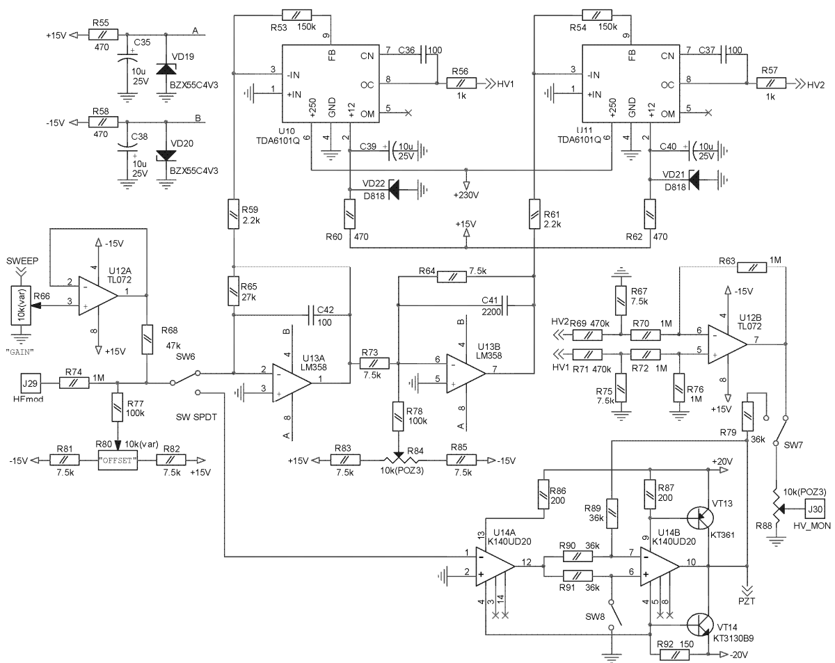
Рис.12. Схема высоковольтного усилителя.
