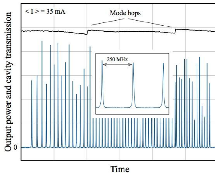
Рис. 4. Зависимость выходной мощности лазера от напряжения на пьезоэлементе (верхняя черная кривая) при постоянном токе LD. Внизу (синяя кривая) – пропускание конфокального интерферометра при тех же условиях. На врезке показан участок, соответствующий перестройке частоты ECDL на 0,6 ГГц.
