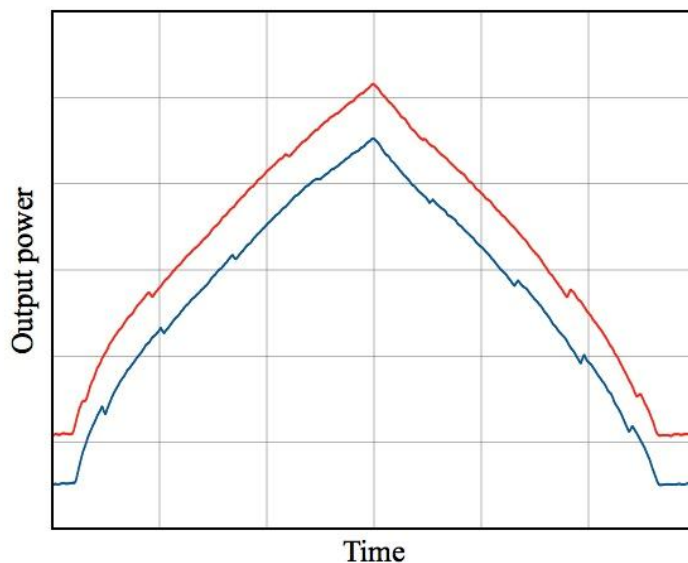
Рис. 5. ВtAX ECDL-6715R при сканировании только тока накачки (синяя кривая) и при сканировании тока накачки вместе с напряжением на пьезоэлементе (красная кривая).
