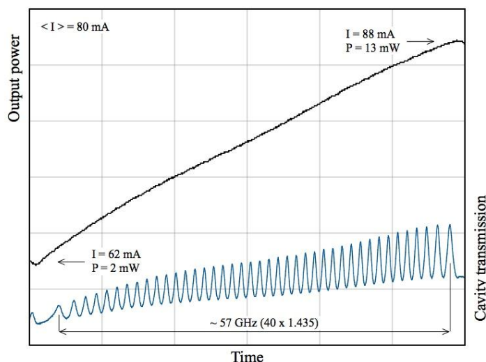
Рис.5. Зависимость мощности ECDL-4210R (верхняя кривая) и пропускание эталона (нижняя кривая) при синхронном сканировании пьезоэлемента и тока накачки.
