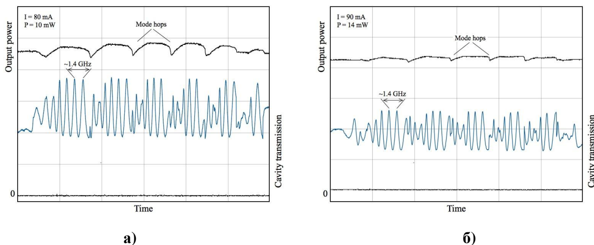
Рис.4. Зависимости выходной мощности лазера от напряжения на пьезоэлементе при постоянном токе LD (верхние черные кривые). Внизу – пропускание эталона Фабри-Перо с областью свободной дисперсии 1.435 ГГц.
