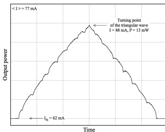
Рис.3. Зависимость выходной мощности лазера от тока инжекции. Ток лазерного диода модулируется симметричным треугольным сигналом. Зависимость снята при постоянном напряжении на пьезоэлементе.
