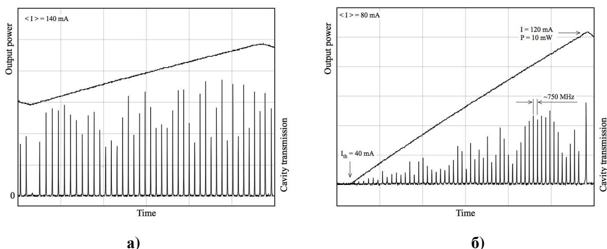
Рис.5. Зависимость мощности ECDL-15510R (верхняя кривая) и пропускание конфокального интерферометра (нижняя кривая) при синхронном сканировании пьезоэлемента и тока накачки (флуктуации амплитуды резонансов связаны с оцифровкой сигнала).
