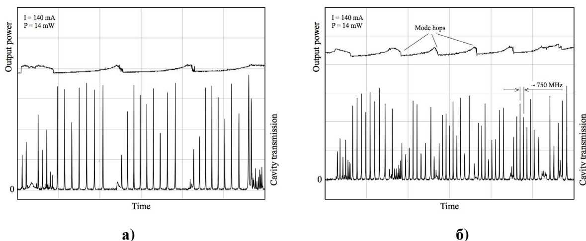
Рис.4. Зависимость выходной мощности лазера от напряжения на пьезоэлементе при постоянном токе LD (верхняя кривая). Внизу – пропускание конфокального интерферометра Фабри-Перо (FSR=750 МГц, флуктуации амплитуды резонансов в области непрерывной перестройки частоты связаны с оцифровкой сигнала).
